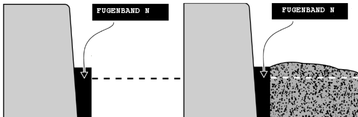
начало укладки ленты
